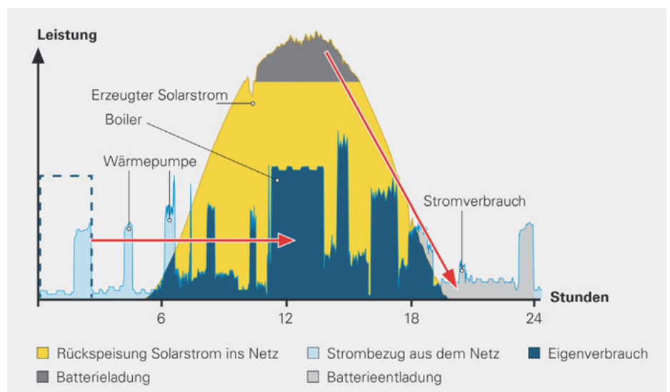
Die intelligente Steuerung managt die Energieverbräuche und optimiert die Stromkosten. Der Ladezyklus des Boilers wird in die Mittagsstunden verschoben und der PV-Peak wird in einer Batterie gespeichert.
